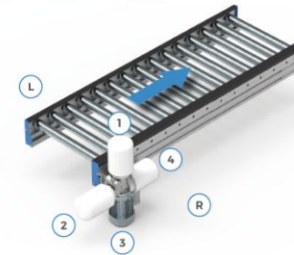
Motorisation directe
